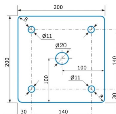
príruba KS420 R = 5mm montážne otvory majú priemer 11mm
